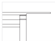
front elevation edge detail
